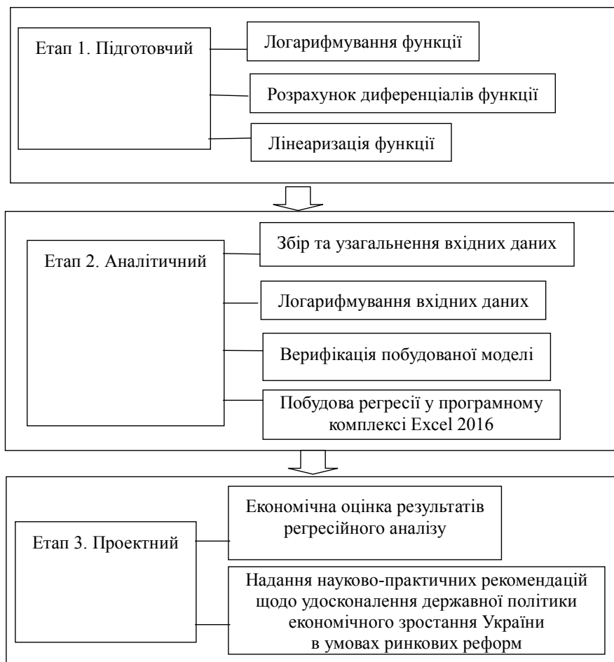
Рис. 1. Послідовність етапів дослідження впливу факторів накопичення на динаміку економічного зростання України в умовах ринкових реформ за допомогою виробничої функції Кобба-Дугласа
