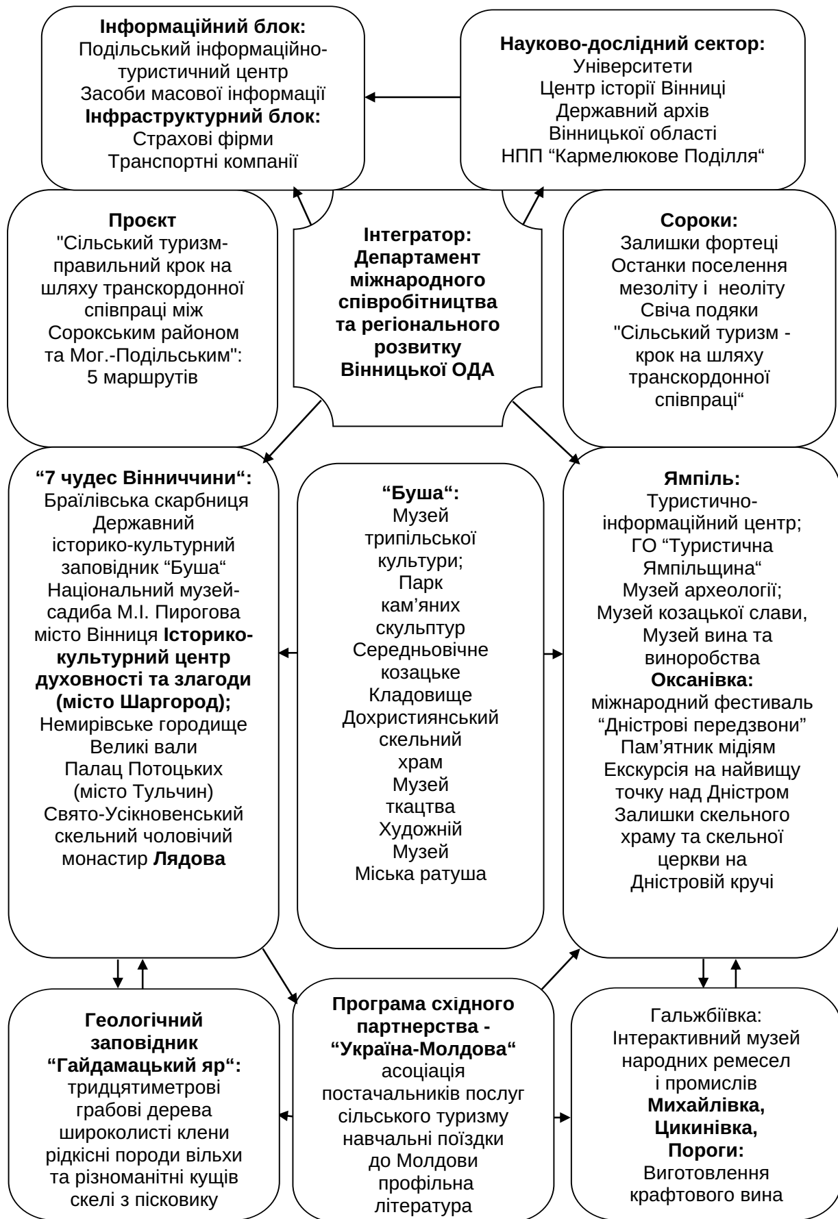
Рис. 3. Модель взаємовідносин у транскордонному кластері
