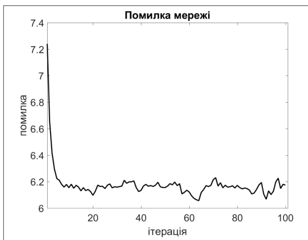
Рис. 4. Зниження помилки нейронної мережі топології 6 x 10 x 1
