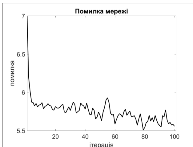
Рис. 3. Зниження помилки нейронної мережі топології 6 x 4 x 1
